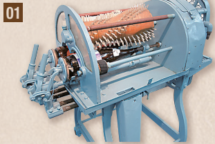
01 二連式壺洗機 (昭和28年) 二本の一升瓶を同時に洗浄でき、当時は手洗いであった壺の洗浄作業の効率化に大きく貢献しました。
