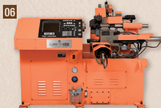
06 CRT付対話型 CNC旋盤 TCC-8 (昭和51年) 機械と人がコミュニケーションできる、国内初のマイクロコンピュータ搭載のCNC (コンピュータ数値制御) 旋盤。
