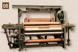
08 K型織機 (昭和35年) 昭和6年から50年間で9万台を製造しました。軽目羽二重から重目織物まで幅広い対応が可能です。
