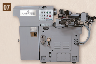
07 精密油圧自動旋盤メリター (昭和49年) 機械と電気制御の一体化により、正確かつ迅速な量産加工と最大240種類の多様な加工が可能です。
