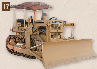
17 D50A ブルドーザ実験車 (昭和36年) 海外資本の自由化対策に対応するため、性能・耐久性の画期的向上を追求した実験車です。
