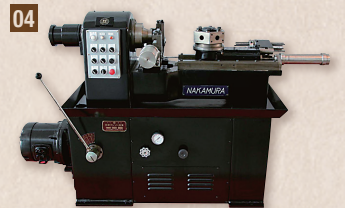
04 油圧自動タレット旋盤 NT5 型 (昭和38年) 油圧と電気制御の組み合わせにより、多くの行程を自動化。簡単かつ多種の加工を可能にしました。
