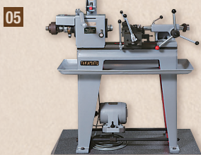
05 面取旋盤 T-650 (昭和39年) 大型旋盤が主流の中、小さな加工品は小さな旋盤でとの発想から開発された省スペース・ローコスト旋盤。
